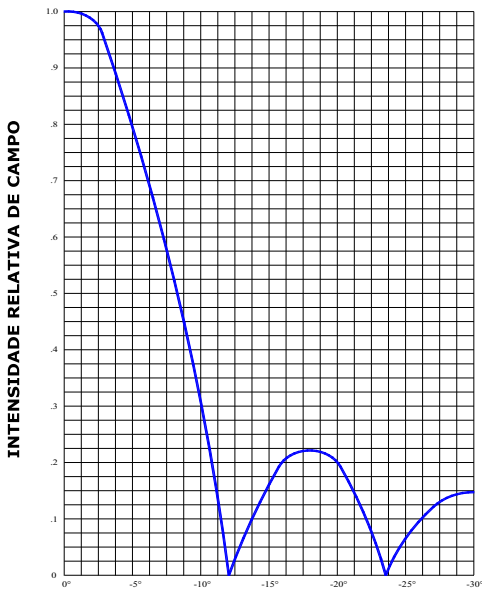
DIAGRAMA DE RADIAÇÃO VERTICAL Escala E/E max 5 Elementos
