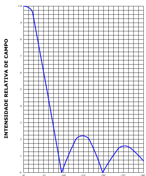
DIAGRAMA DE RADIAÇÃO VERTICAL Escala E/E max 6 Elementos
