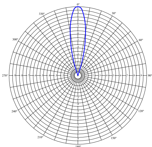
DIAGRAMA DE RADIAÇÃO HORIZONTAL Escala E/Emax
