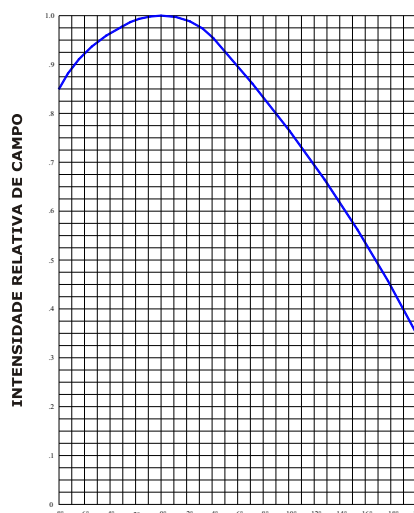
DIAGRAMA DE RADIAÇÃO VERTICAL Escala E/Emax
